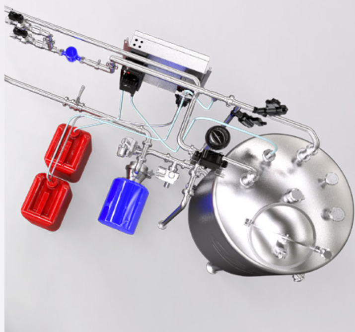
Dettaglio: sistema di pompaggio completamente automatizzato
